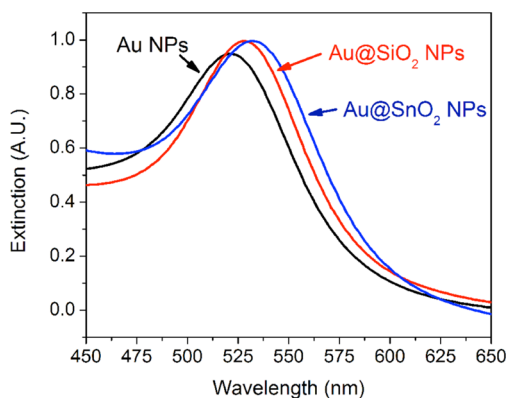
Figure 2. Extinction spectra of citrate-stabilized Au nanoparticles (Au NPs), SiO 2 -coated Au nanoparticles (Au@SiO 2 NPs), and SnO 2 -coated Au nanoparticles (Au@SnO 2 NPs).
